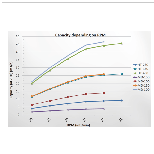
Kapacitetsdiagram för rotorlussar HT/HT-S/MD
