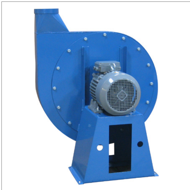
HV - Högtrycksfläkt för renluft
